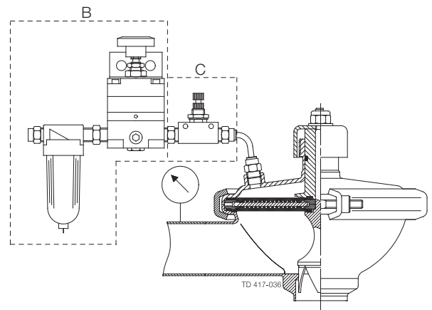
Fig. 2. CPMI-2 con válvula reguladora de presión y calibrador de presión.
